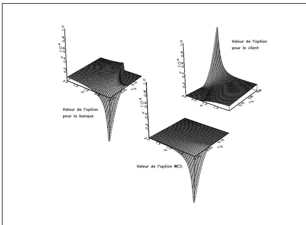
FIG. 27: Influence du paramètre a sur la valeur des options
