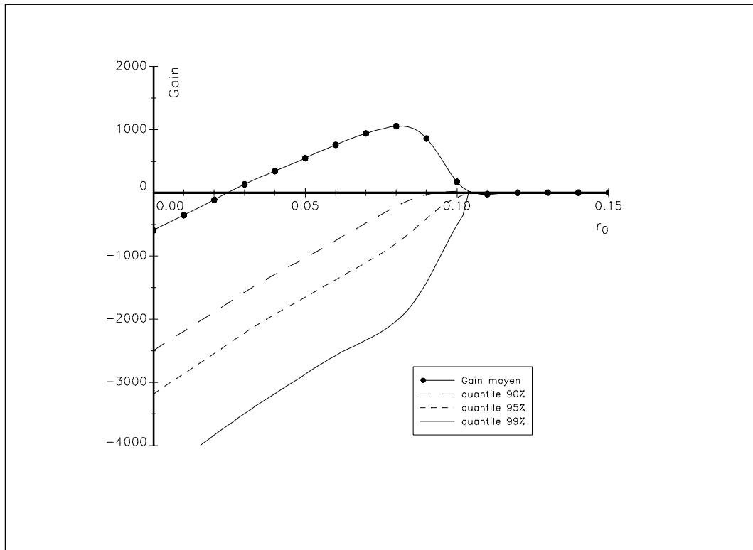
FIG. 12: Quantiles de la distribution
