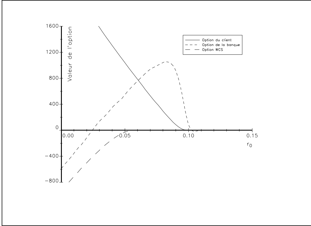
FIG. 9: Pire scénario pour la banque
