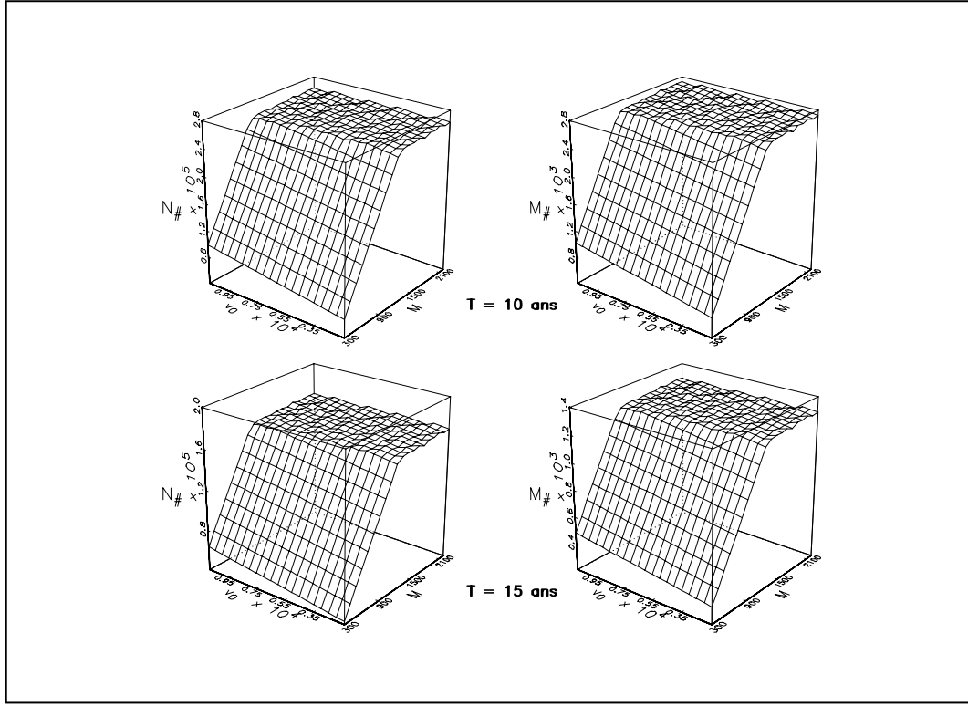
FIG. 5: Mensualité M_{\#} et nominal N_{\#} au moment où la prime d'état est saturée
