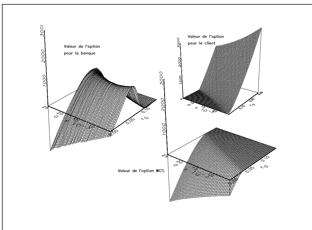
FIG. 29: Influence du paramètre \sigma sur la valeur des options
