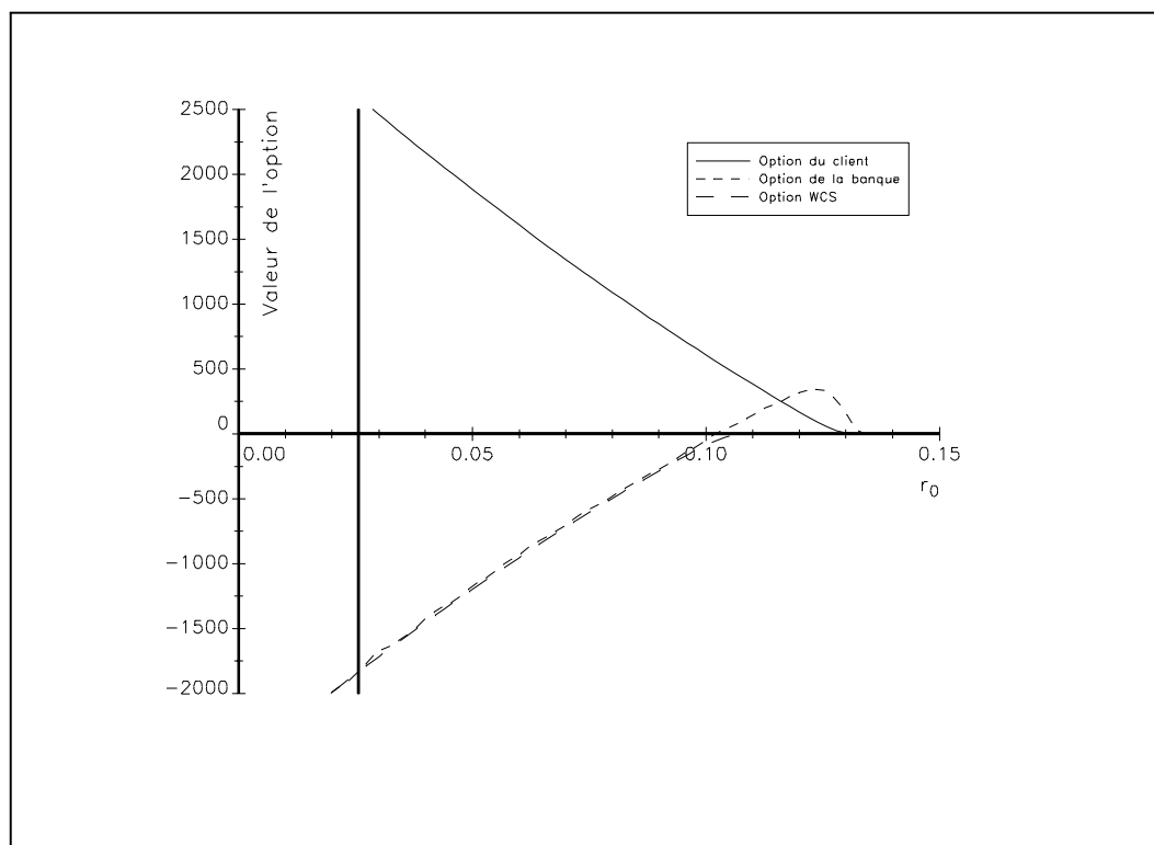
FIG. 19: Influence du mode de calcul des droits à prêts sur la valeur des options
