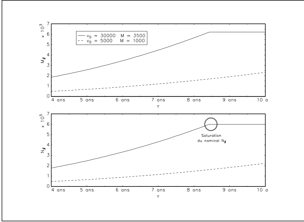
FIG. 1: Influence du temps de conversion sur la mensualité et le nominal du crédit
