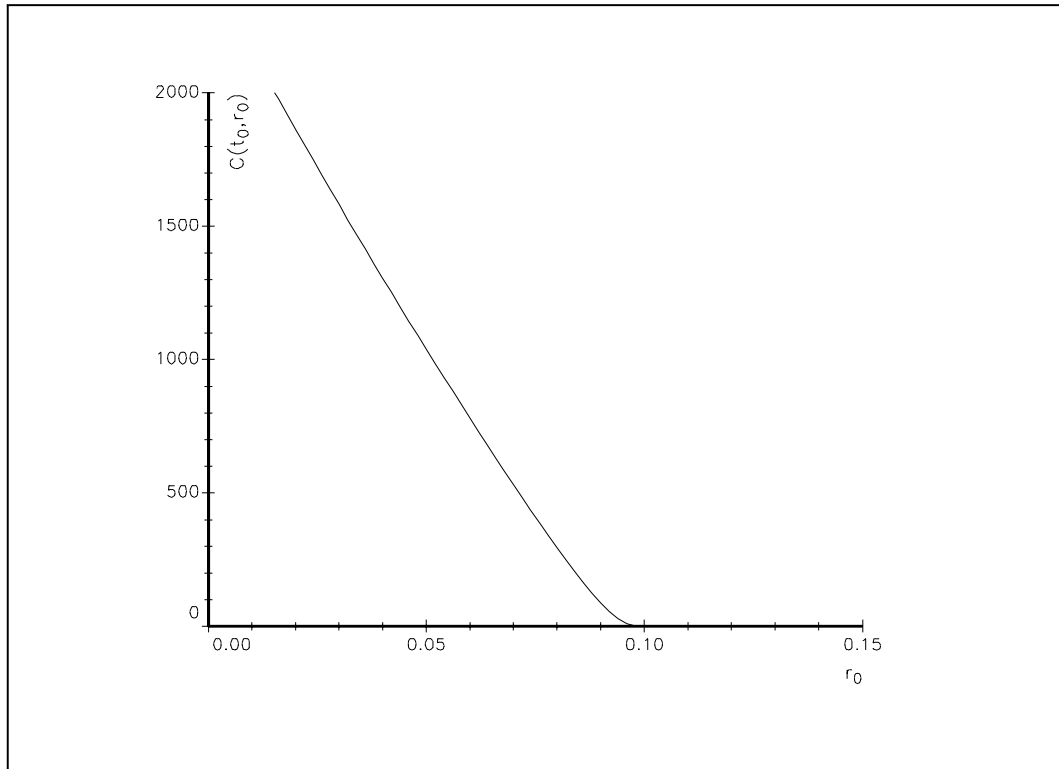
FIG. 6: Valeur de l'option C(t_0, r_0) pour le détenteur du PEL
