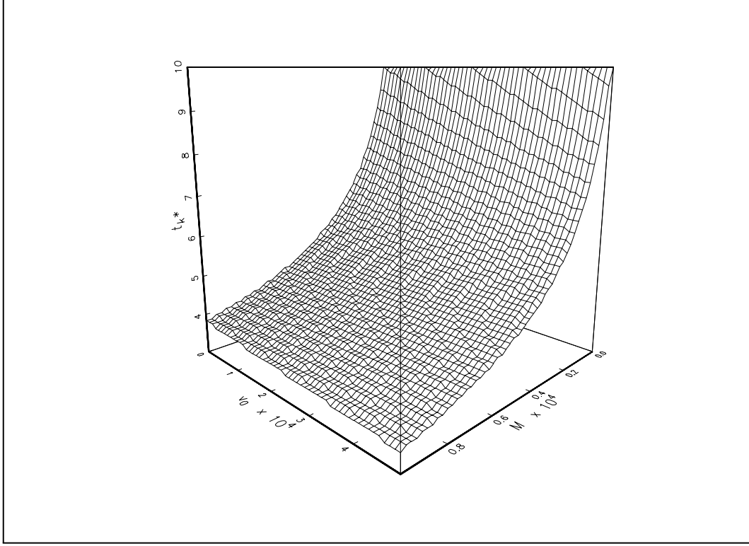
FIG. 2: Temps t_{k^*} (en année) nécessaire pour saturer la prime d'état
