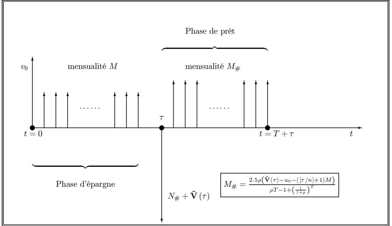
FIG. 3: Échéancier aléatoire du PEL (phases de prêt et d'emprunt)
