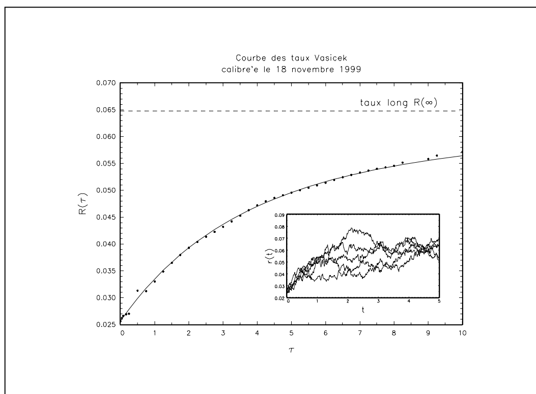
FIG. 14: Courbe des taux du 18 novembre 1999
