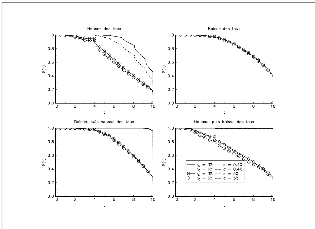
FIG. 26: Fonctions de survie
