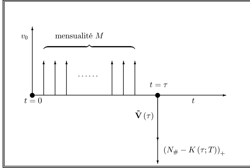
FIG. 4: Échéancier associé à C(t_0)
