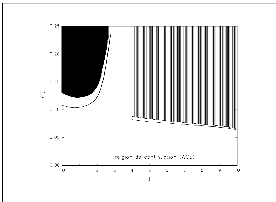
FIG. 20: Influence du mode de calcul des droits à prêts sur les frontières d'exercice
