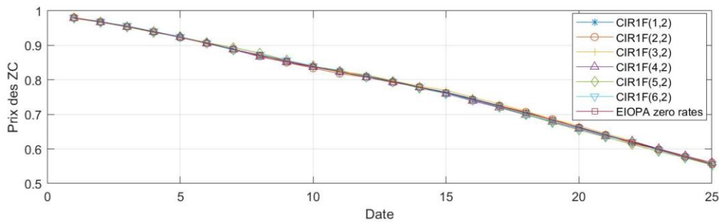
Figure 3 : test 3 - convergence des ZC 10 ans déflatés vers les prix observés du marché : E^P(D(t) * P(t, t + 10)) = P^M(0, t + 10)
