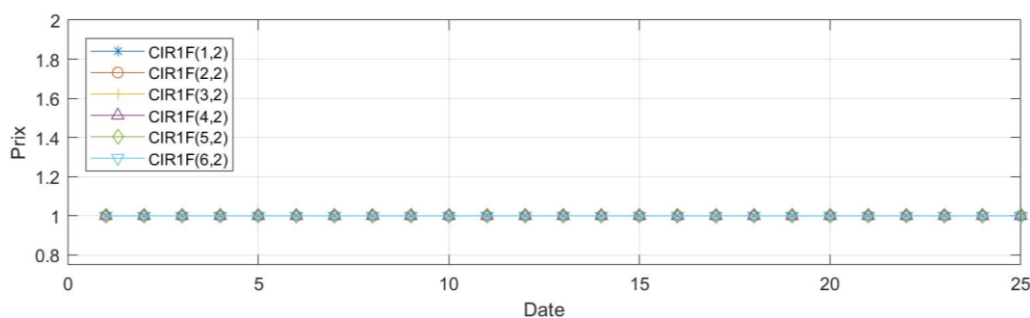
Figure 5 : test 5 - martingalité de l'actif risqué : E^P(D(t).S(t)) = S(0)
