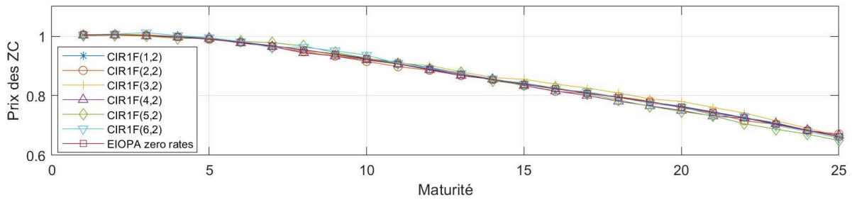
Figure 2 : test 2 - convergence des ZC 5 ans déflatés vers les prix observés du marché : E^P(D(t) * P(t, t + 5)) = P^M(0, t + 5)
