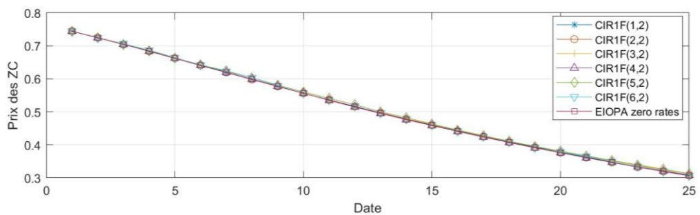
Figure 4 : test 4 - convergence des ZC 20 ans déflatés vers les prix observés du marché : E^P(D(t) * P(t, t + 20)) = P^M(0, t + 20)
