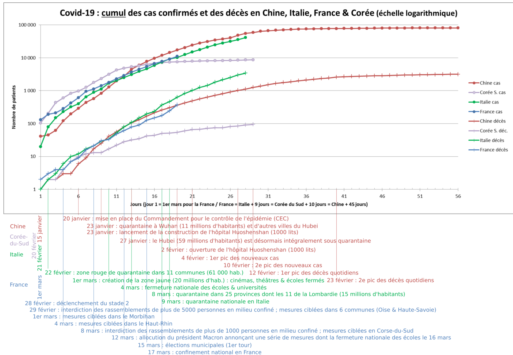
Figure 1 : cumul des cas et des décès en échelle logarithmique (Chine, Corée du Sud, Italie et France)
